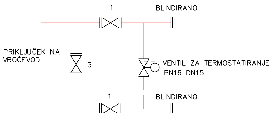
15/2: VGRADNJA TERMOSTATIRANE KRATKE VEZI ZARADI VAROVANJA PRED ZMRZOVANJEM (ZAČASNO ODKLOPLJENI OBJEKTI)
